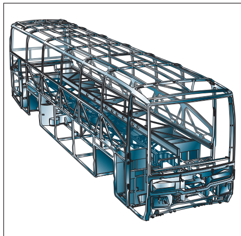
Рис. 7.5. Несущая конструкция кузова автобуса
