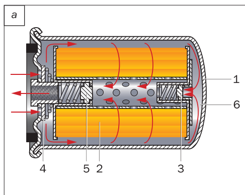
Рис. 2.45. Устройство неразборного (а) и разборного (б) полнопоточного объемно-адсорбирующего масляного фильтра: 1 — корпус; 2 — штора (фильтрующий элемент); 3 — перепускной клапан; 4 — противодренажный клапан; 5 — противосливной клапан; 6 — путь масла при открытии перепускного клапана; 7 — канал слива масла в картер при замене фильтрующего элемента
