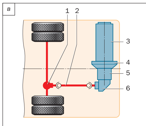
Рис. 1.26. Заднеприводная заднемоторная компоновка с поперечным расположением двигателя и углом \beta равным 60^\circ (а), 80^\circ (б) и 90^\circ (в): 1 — главная передача; 2 — карданная передача; 3 — двигатель; 4 — сцепление; 5 — коробка передач; 6 — угловой редуктор
