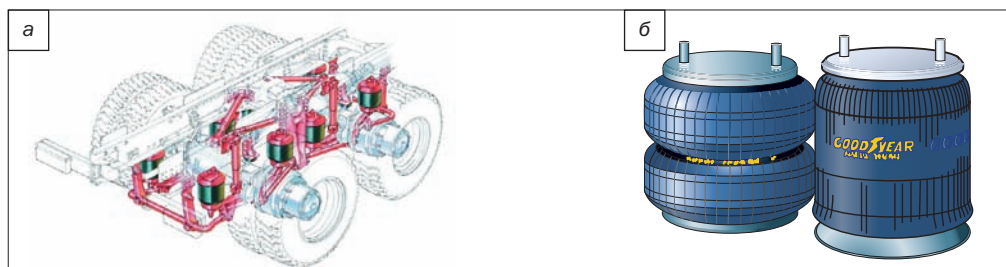
Рис. 4.29. Упругие элементы пневматических подвесок: а — рукавного типа; б — двойные баллоны
