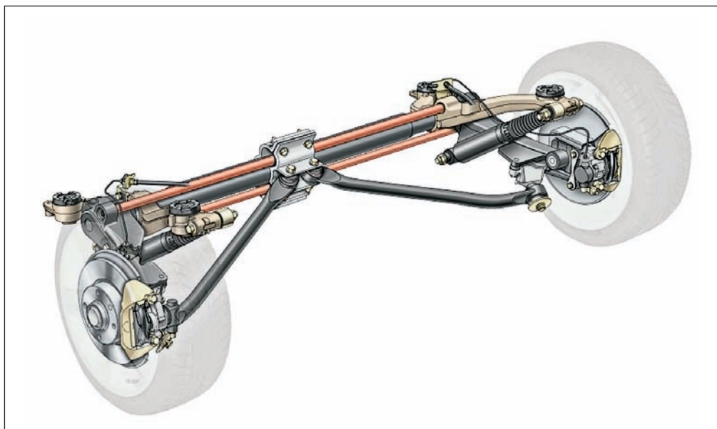
Рис. 4.28. Тормсионная подвеска. В задней подвеске автомобиля Peugeot 206 используются два торсиона, соединенные с продольными рычагами. В направляющем устройстве подвески применяются трубчатые рычаги, установленные под углом к продольной оси автомобиля
