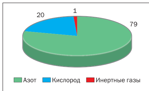
Рис. 2.57. Состав воздуха, %
