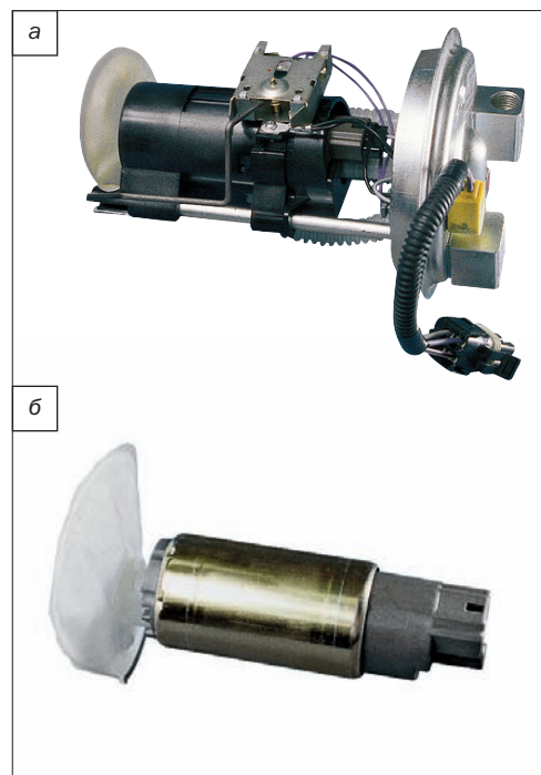
Рис. 2.66. Погружной электрический топливный насос: а — топливозаборник с насосом; б — внешний вид насоса; варианты исполнения насосной секции: в — шестеренчатая; г — роликковая; д — пластинчатая; е — схема работы насосной секции роторного типа (1 — корпус; 2 — зона всасывания; 3 — ротор; 4 — зона нагнетания; 5 — направление вращения)
