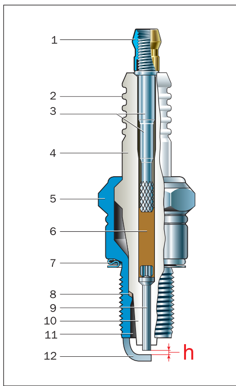
Рис. 2.113. Свеча зажигания бензинового двигателя: 1 — контактная гайка; 2 — ребрение изолятора (барьеры для тока утечки); 3 — контактный стержень; 4 — керамический изолятор; 5 — металлический корпус; 6 — токопроводящий стеклогерметик; 7 — уплотнительное кольцо; 8 — теплоотводящая шайба; 9 — центральный электрод; 10 — тепловой конус изолятора; 11 — рабочая камера; 12 — боковой электрод «масса»; h — искровой зазор
