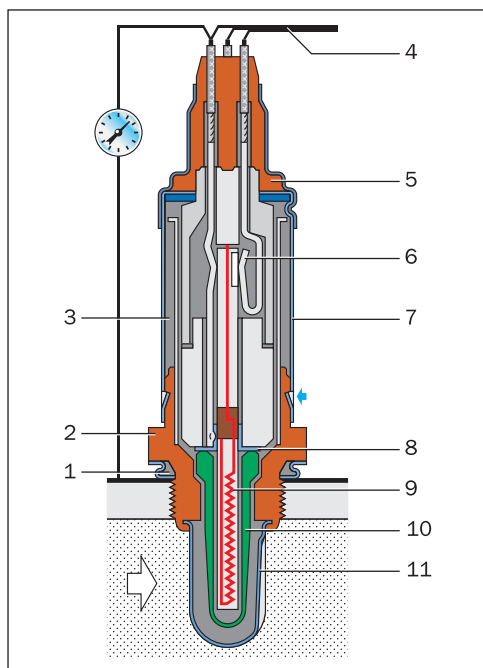
Рис. 2.77. Устройство датчика концентрации кислорода: 1 — уплотнительное кольцо; 2 — металлический корпус с резьбой и шестигранником «под ключ»; 3 — керамический изолятор; 4 — провода; 5 — уплотнительная манжета проводов; 6 — токоподводящий контакт провода питания нагревателя; 7 — наружный защитный экран с отверстием для атмосферного воздуха; 8 — токоотъемник электрического сигнала; 9 — электрический нагреватель; 10 — керамический наконечник; 11 — защитный экран с отверстием для отработавших газов
