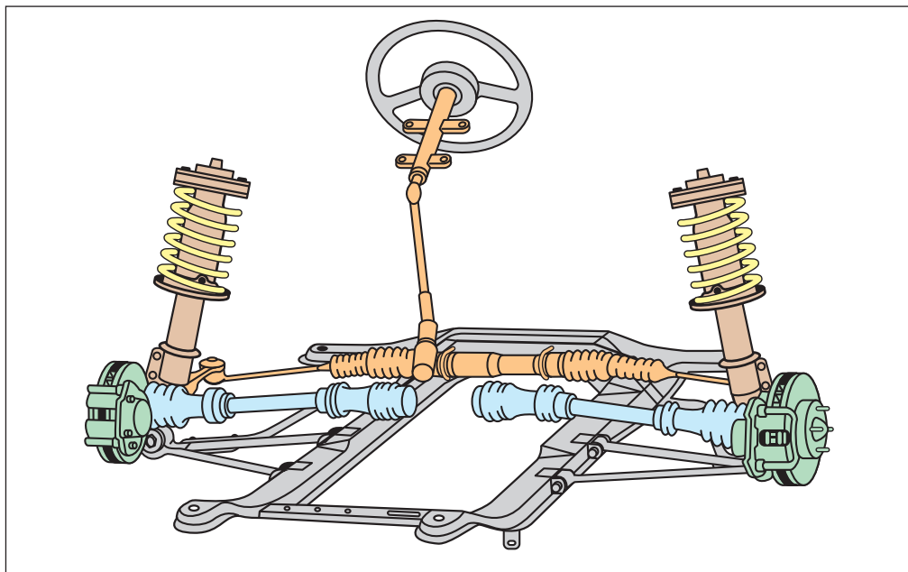
Рис. 4.42. Схема подвески Мак-Ферсон
