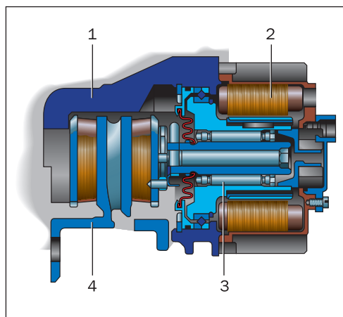
Рис. 6.9. Дисковый тормозной механизм с электрическим приводом: 1 — скоба; 2 — обмотка; 3 — шток; 4 — тормозной диск
