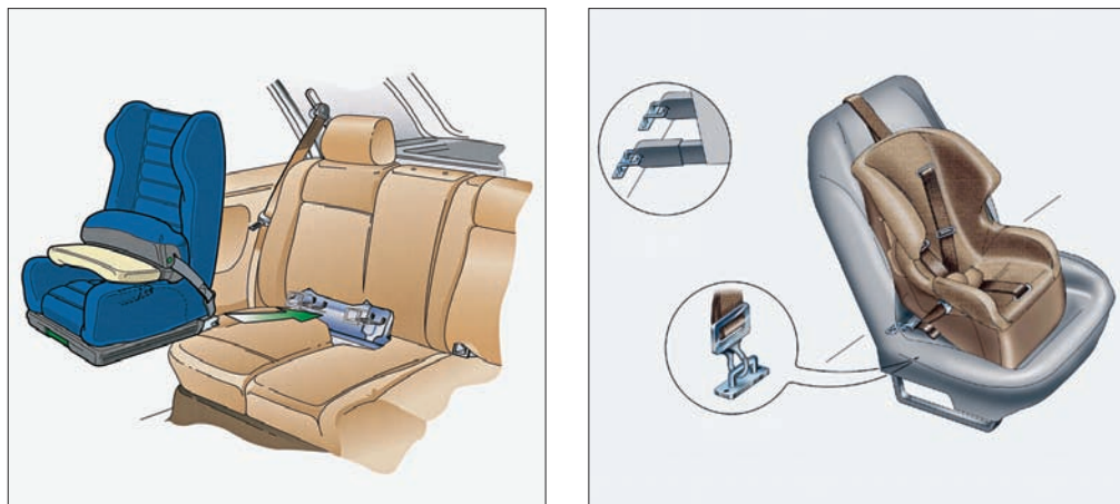
Рис. 7.26. Варианты крепления детских сидений по стандарту ISOFIX
