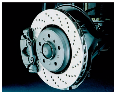
Рис. 6.11. Тормозной механизм с вентилируемым диском
