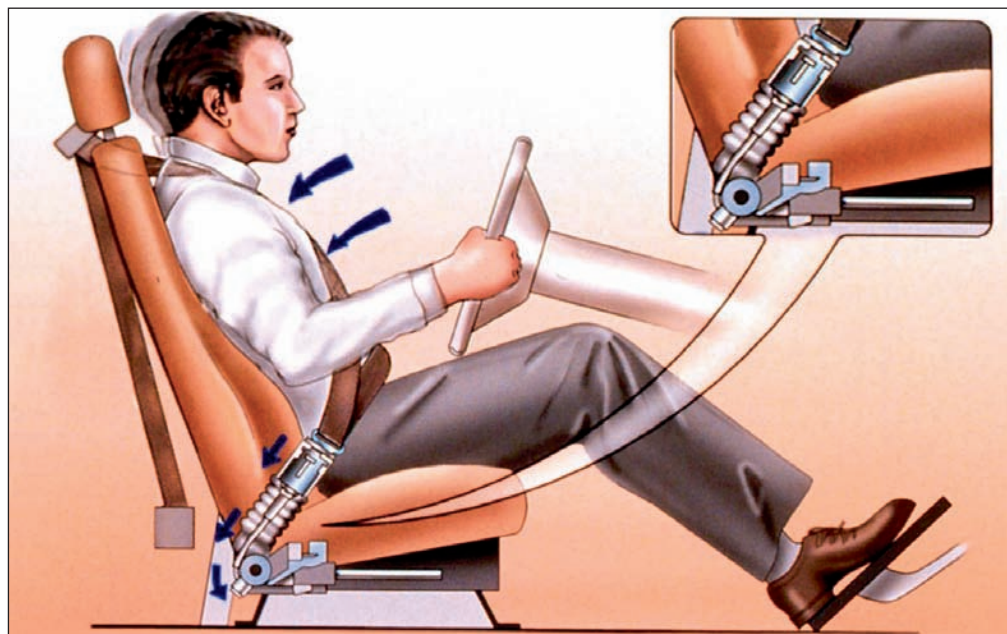
Рис. 7.23. Схема крепления ремня безопасности с преднатяжителем
