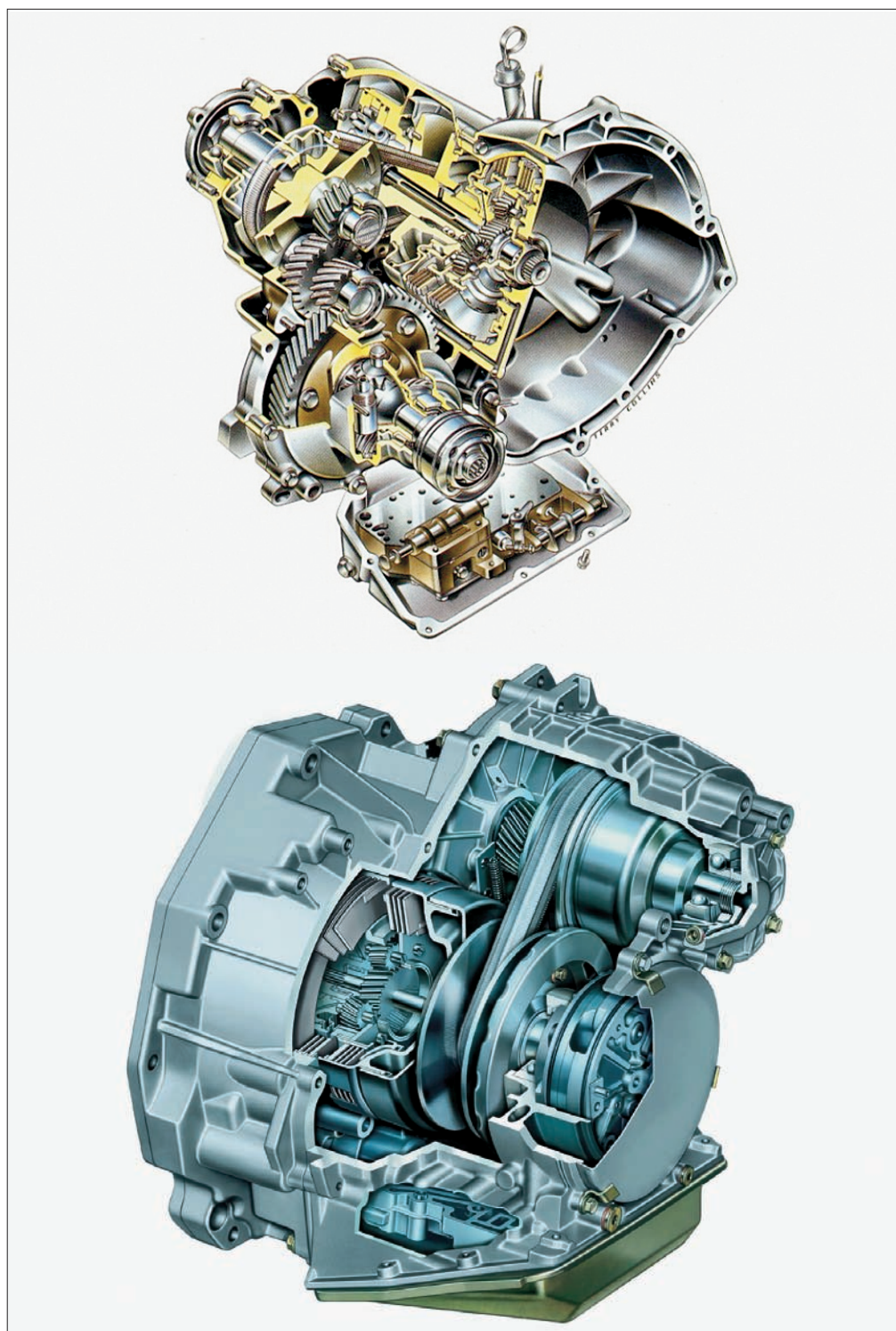
Рис. 3.44. Коробка передач Hyper CVT-M6
