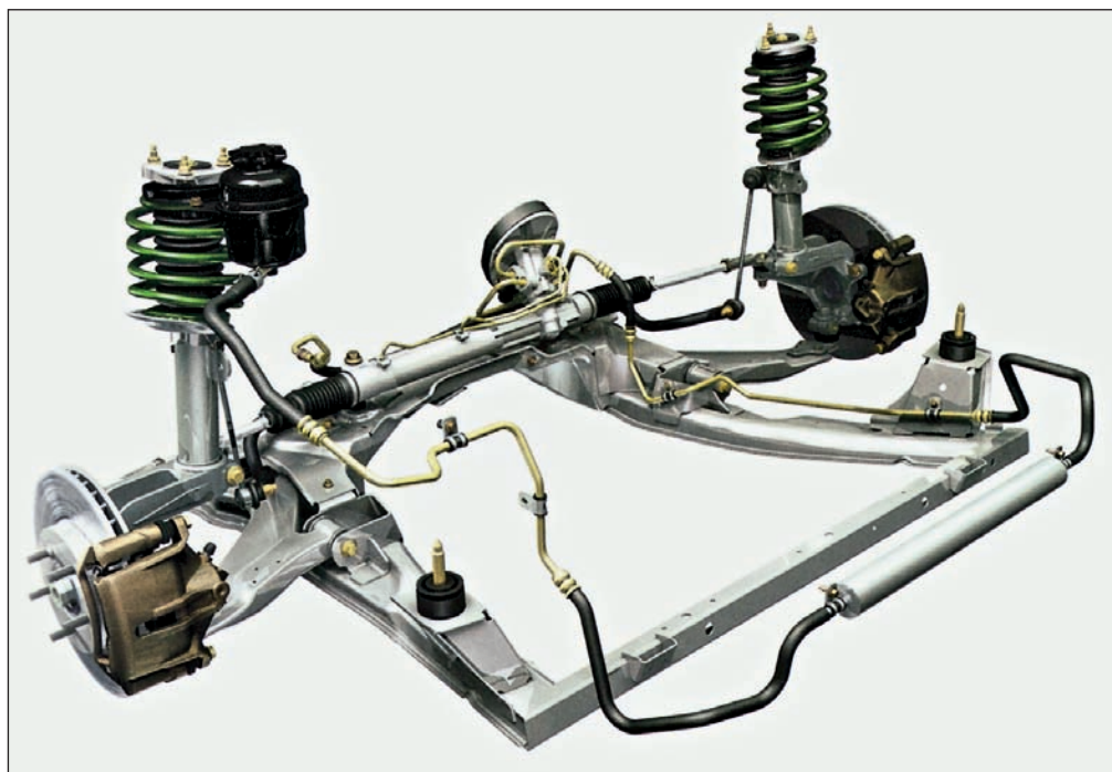
Рис. 4.57. Управляемый мост
