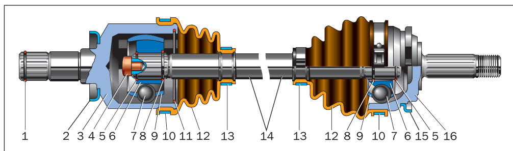
Рис. 3.25. Шестишариковые шарниры равных угловых скоростей: 1 — стопорное кольцо корпуса внутреннего шарнира; 2 — защитное кольцо внутреннего шарнира; 3 — корпус внутреннего шарнира; 4 — упор вала; 5 — стопорное кольцо; 6 — обойма; 7 — шарик; 8 — упорное кольцо; 9 — сепаратор; 10 — наружный хомут; 11 — фиксатор внутреннего шарнира; 12 — защитный чехол; 13 — внутренний хомут; 14 — вал привода колеса; 15 — защитное кольцо наружного шарнира; 16 — корпус наружного шарнира
