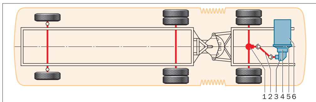
Рис. 1.29. Сочлененный автобус с толкающей задней секцией с поперечным расположением двигателя в задней прицепной секции: 1 — главная передача; 2 — карданная передача; 3 — угловой редуктор; 4 — коробка передач; 5 — сцепление; 6 — двигатель
