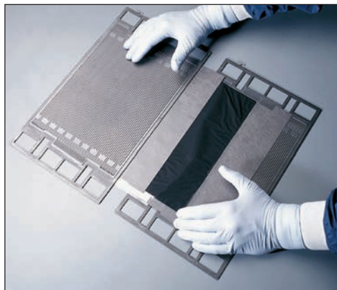
Рис. 8.11. Отдельная ячейка топливного элемента
