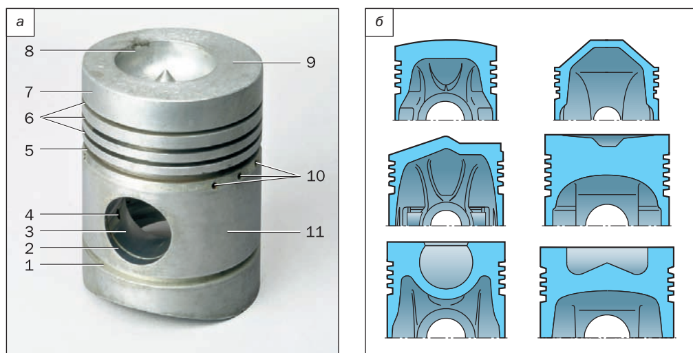
Рис. 2.23. Поршень дизельного двигателя (а) грузового автомобиля и формы поршней разных двигателей (б): 1 — канавка нижнего маслосъемного кольца; 2 — проточка под стопорное кольцо поршневого пальца; 3 — внутренняя поверхность бобышки; 4 — отверстие для смазки поршневого пальца; 5 — канавка верхнего маслосъемного кольца; 6 — канавки компрессионных колец; 7 — головка поршня; 8 — камера сгорания в поршне; 9 — днище поршня; 10 — отверстия для отвода масла; 11 — юбка
