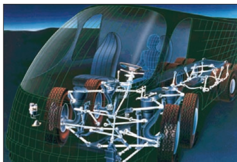
Рис. 5.10. Рулевой привод многоосных автомобилей
