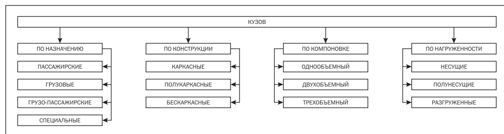
Рис. 7.2. Классификация кузовов
