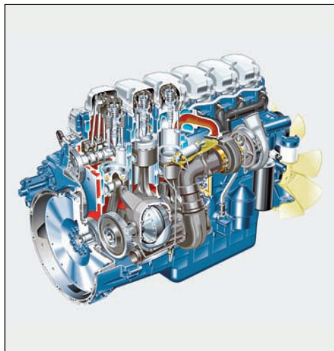
Рис. 2.110. Турбокомпаундный двигатель Scania
