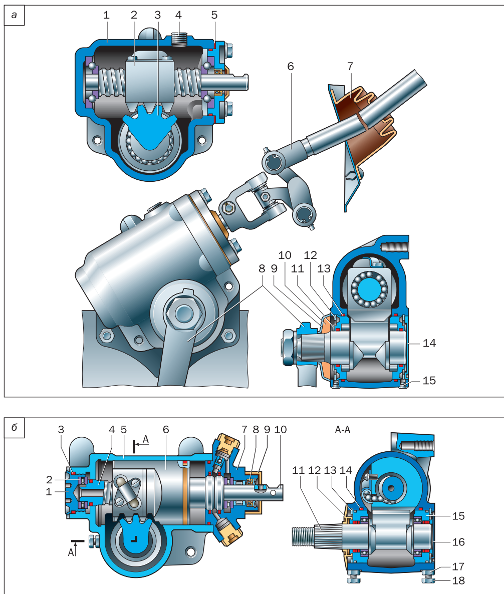
Рис. 5.8. Рулевой механизм типа «винт-шариковая гайка–рейка–зубчатый сектор» без гидроусилителя (а): 1 — картер; 2 — винт с шариковой гайкой; 3 — вал-сектор; 4 — пробка заливного отверстия; 5 — регулировочные прокладки; 6 — вал; 7 — уплотнитель рулевого вала; 8 — сошка; 9 — крышка; 10 — уплотнитель вала-сектора; 11 — наружное кольцо подшипника вала-сектора; 12 — стопорное кольцо; 13 — уплотнительное кольцо; 14 — боковая крышка; 15 — пробка; со встроенным гидроусилителем (б): 1 — регулировочная гайка; 2 — подшипник; 3 — уплотнительное кольцо; 4 — винт; 5 — картер; 6 — поршень-рейка; 7 — гидравлический распределитель; 8 — манжета; 9 — уплотнитель; 10 — входной вал; 11 — вал-сектор; 12 — защитная крышка; 13 — стопорное кольцо; 14 — уплотнительное кольцо; 15 — наружное кольцо подшипника вала-сектора; 16 — боковая крышка; 17 — гайка; 18 — болт
