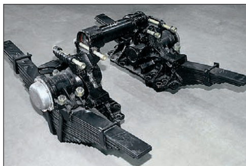
Рис. 4.53. Балансирная подвеска
